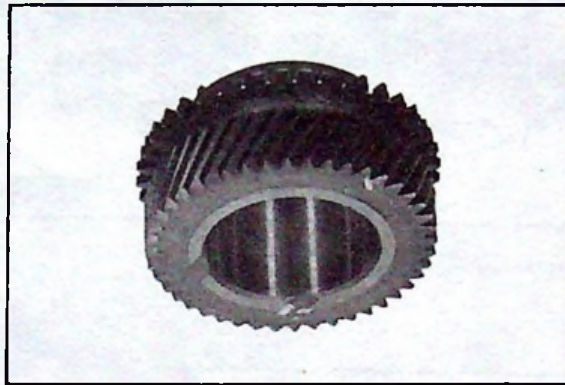
Pignon récepteur de 4ème : ZA. 4 264 743
