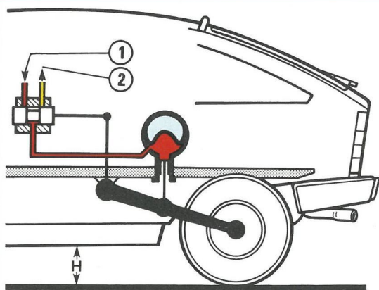
1 - Arrivée de pression 2 - Retour au réservoir
